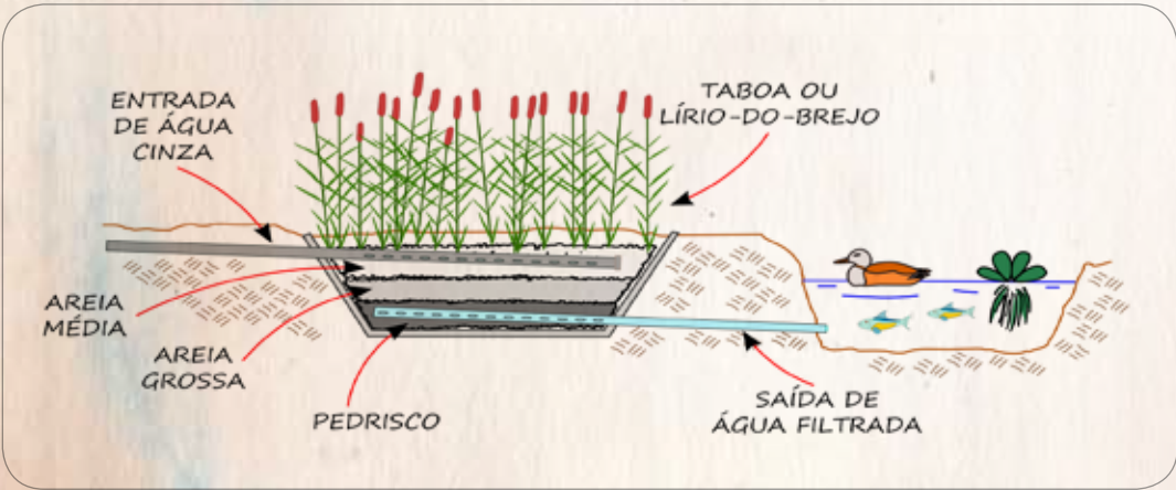
Biofiltro - leito filtrando ou filtro de raízes. Adaptado de OMS. Guía de orientación en Saneamiento Básico. http://www.bvsde.ops-oms.org/bvsacg/guialcalde/2sas/2-4sas.htm
