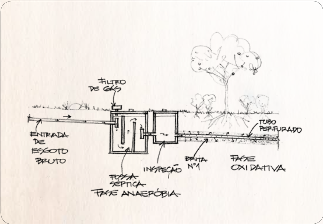
Biofiltro de esgoto - sistema Lavoisier - vala de infiltração subsuperficial. Adaptado do desenho original de Peter Webb.
